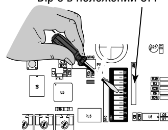
Dip 6 в положении OFF
